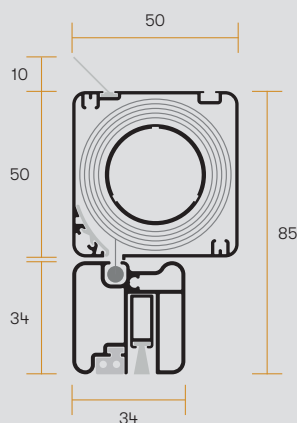
Caisson et barre poignée Box and Handle bar
